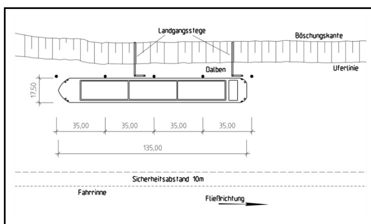
Fig. 1 : Poste de stationnement à ducs d'Albe avec un automoteur à marchandises montant
