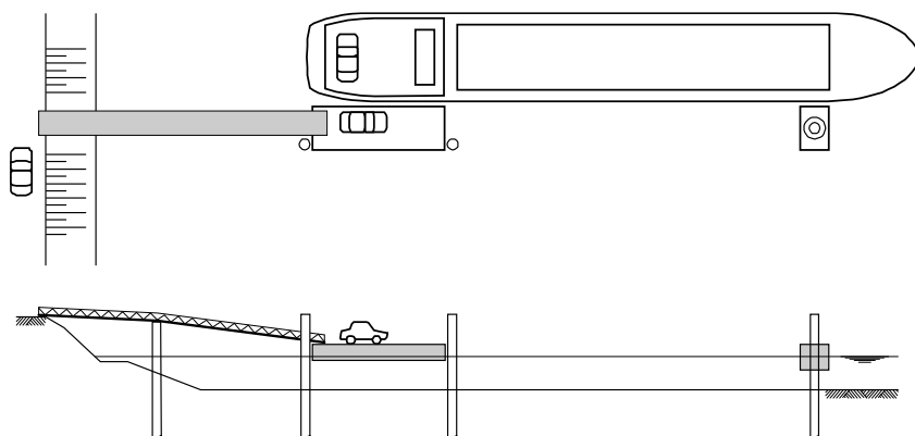
Figure 43: poste de débarquement de véhicules motorisés muni d'un ponton ou d'un débarcadère adapté aux niveaux d'eau variables
