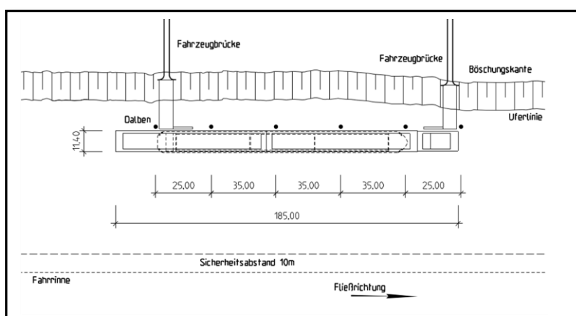
Fig. 5: Emplacement pour la dépose d'automobiles avec 2 ponts pour véhicules
