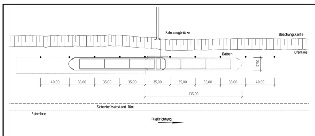
Fig. 4: Emplacement pour la dépose d'automobiles avec 1 pont pour véhicules et des ducs d'Albe en amont et en aval pour l'accostage des montants et avalants.
