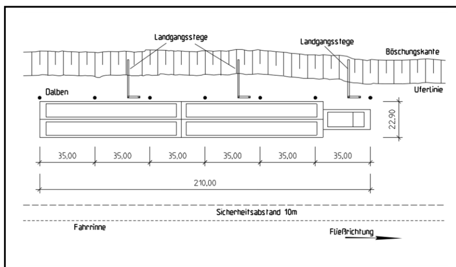
Fig. 3 : Poste de stationnement à ducs d'Albe avec un convoi poussé
