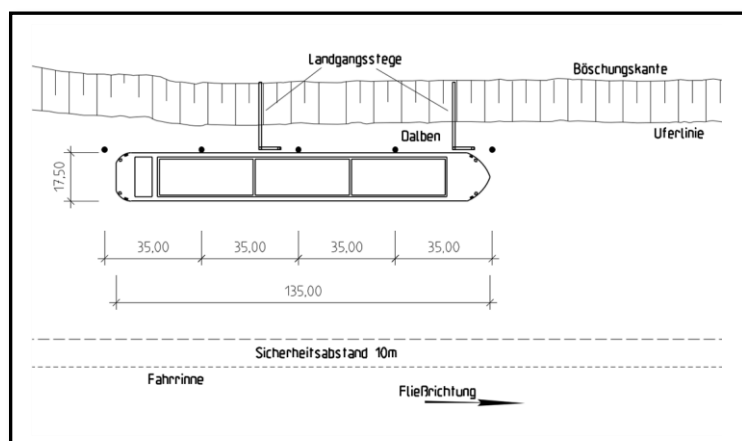
Fig. 2 : Poste de stationnement à ducs d'Albe avec un automoteur à marchandises avalant
