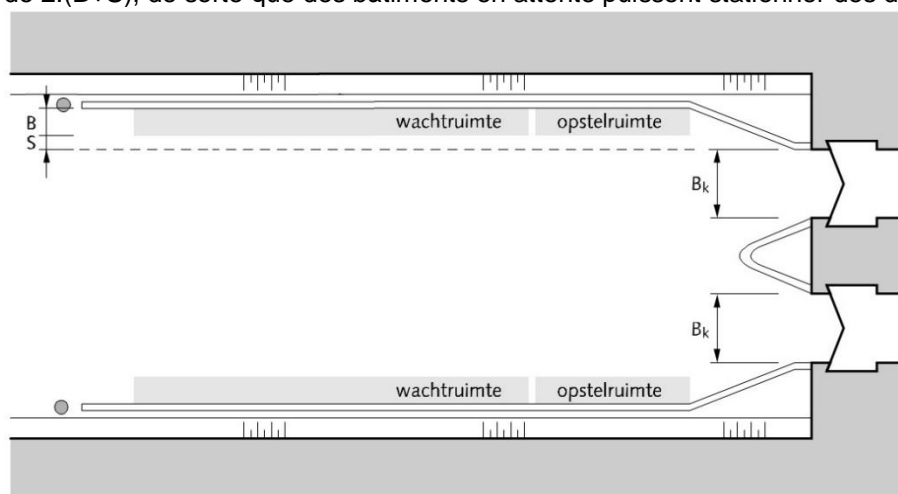
Figure 23 : ensemble d'écluses avec deux sas identiques 12
